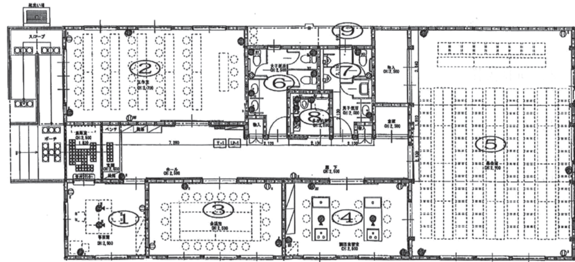
①事務室 ②工作室 ③会議室 ④調理実習室 ⑤集会室 ⑥女子トイレ ⑦男子トイレ ⑧多目的トイレ ⑨発電機
